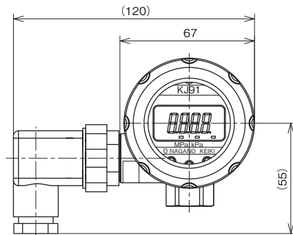
《直結形》電線取出口 左向き
