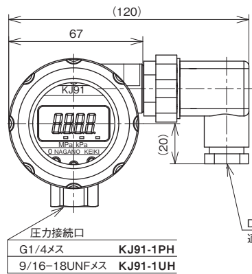
《直結形》電線取出口 右向き
