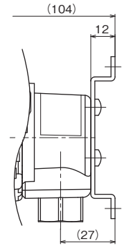
パネル取付形の場合
