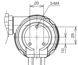
背面図
