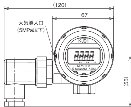
《直結形》電線取出口 左向き
