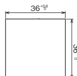
パネルカット寸法
